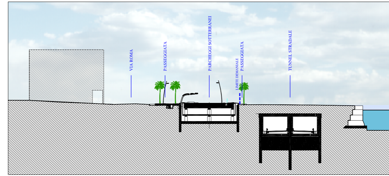
SEZIONI TRASVERSALI TIPICHE 1:1000
