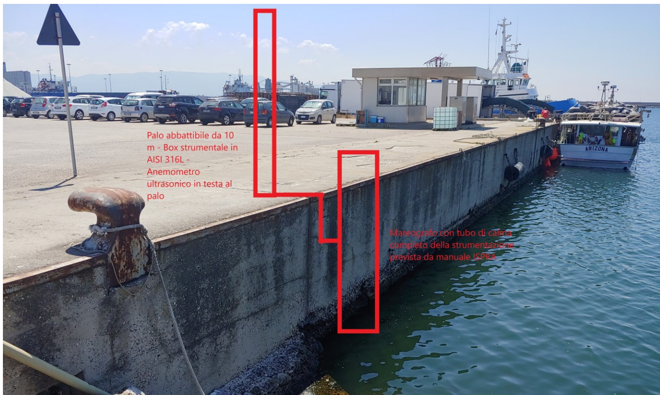
Figura 2 – Indicazioni di installazione
